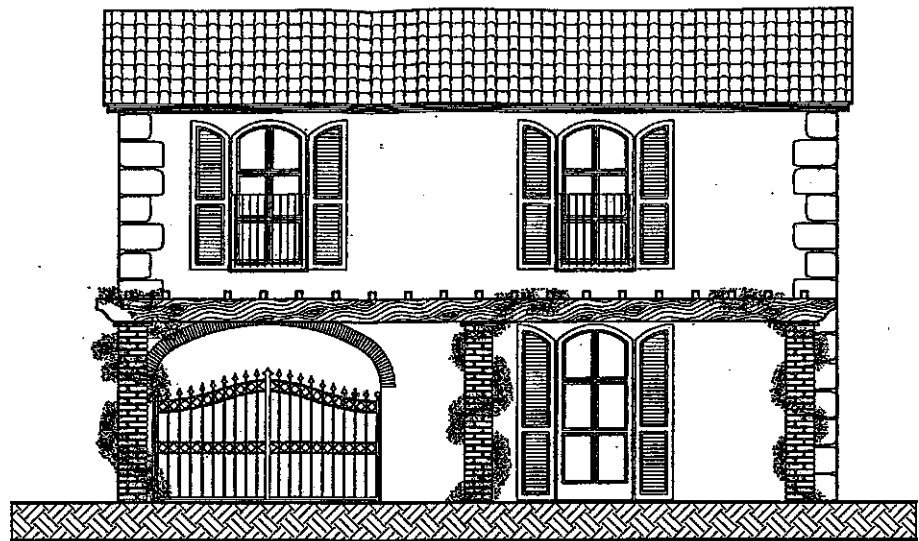
PROSPETTO SUD
