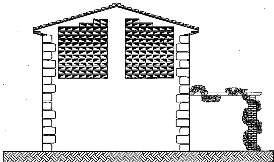
PROSPETTO OVEST
