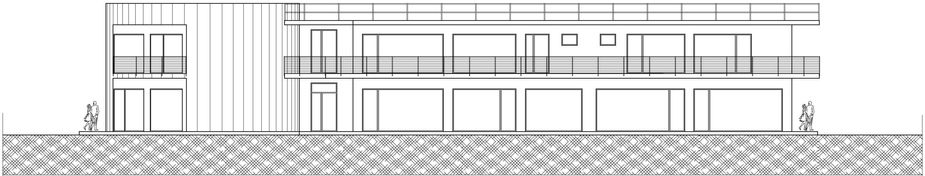
PROSPETTO OVEST
